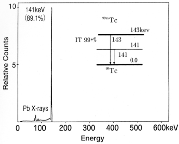
Tc-99m
