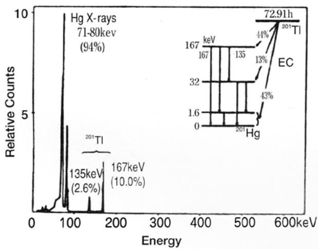
Tl-201
