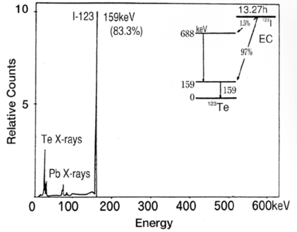
I-123
